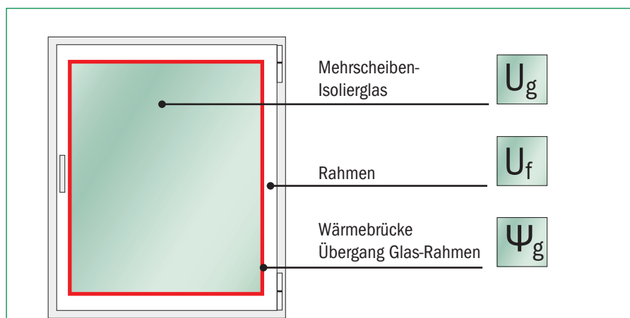
Abb. 10: Der U_w -Wert eines Fensters setzt sich aus zwei flächenbezogenen Wärmedurchgangskoeffizienten U und einem linearen Wärmedurchgangskoeffizienten \Psi zusammen.
