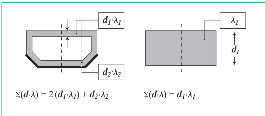
Abb. 5: Ein Abstandhalter ist dann wärmetechnisch verbessert, wenn er das Kriterium \Sigma(d \cdot \lambda) \leq 0,007 erfüllt. Die Abbildung zeigt an zwei Beispielen, wie dieses Merkmal bei Abstandhaltern bestimmt wird [1, 3].
